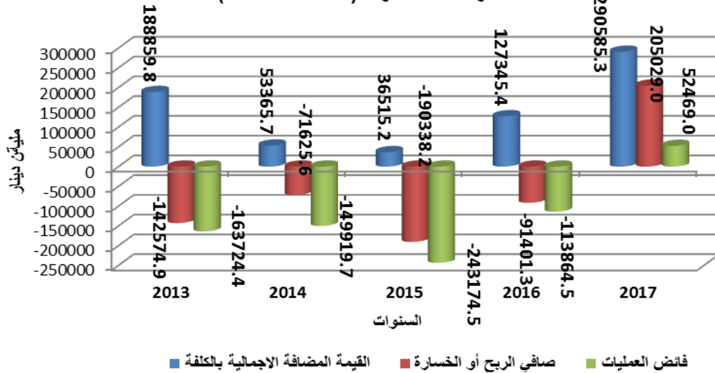
شكل رقم (4) المؤشرات الرئيسية لنشاط صناعة المنتجات المعدنية المصنعة والمكانن والمعدات للسنوات (2017 - 2013)
